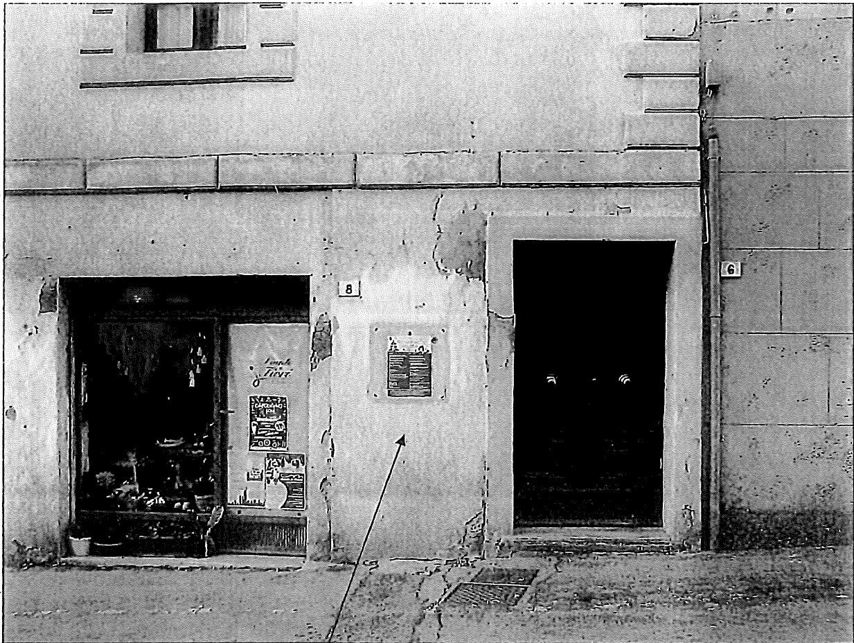
Figura 1 quadro elettrico posizionamento
